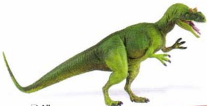
Allosaurus
